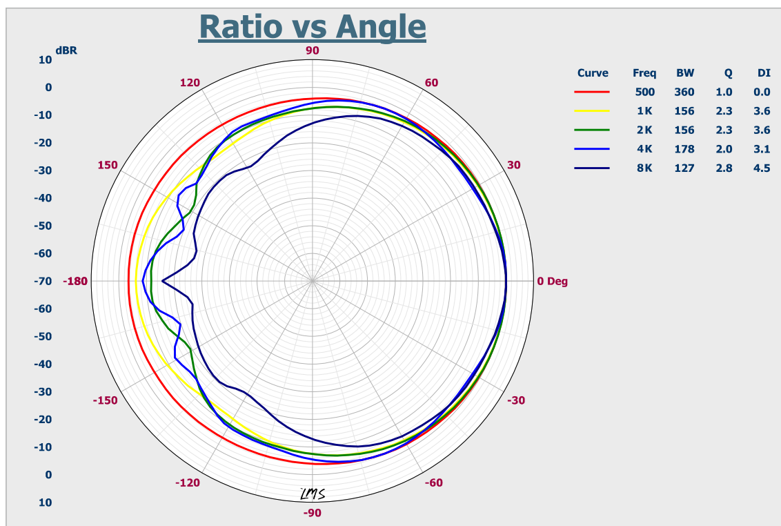
Круговая диаграмма направленности громкоговорителя LPA-MUSIC-30 (цвет черный)
